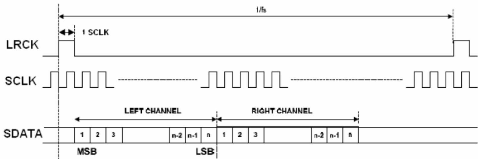
DSP (PCM) Mode A
