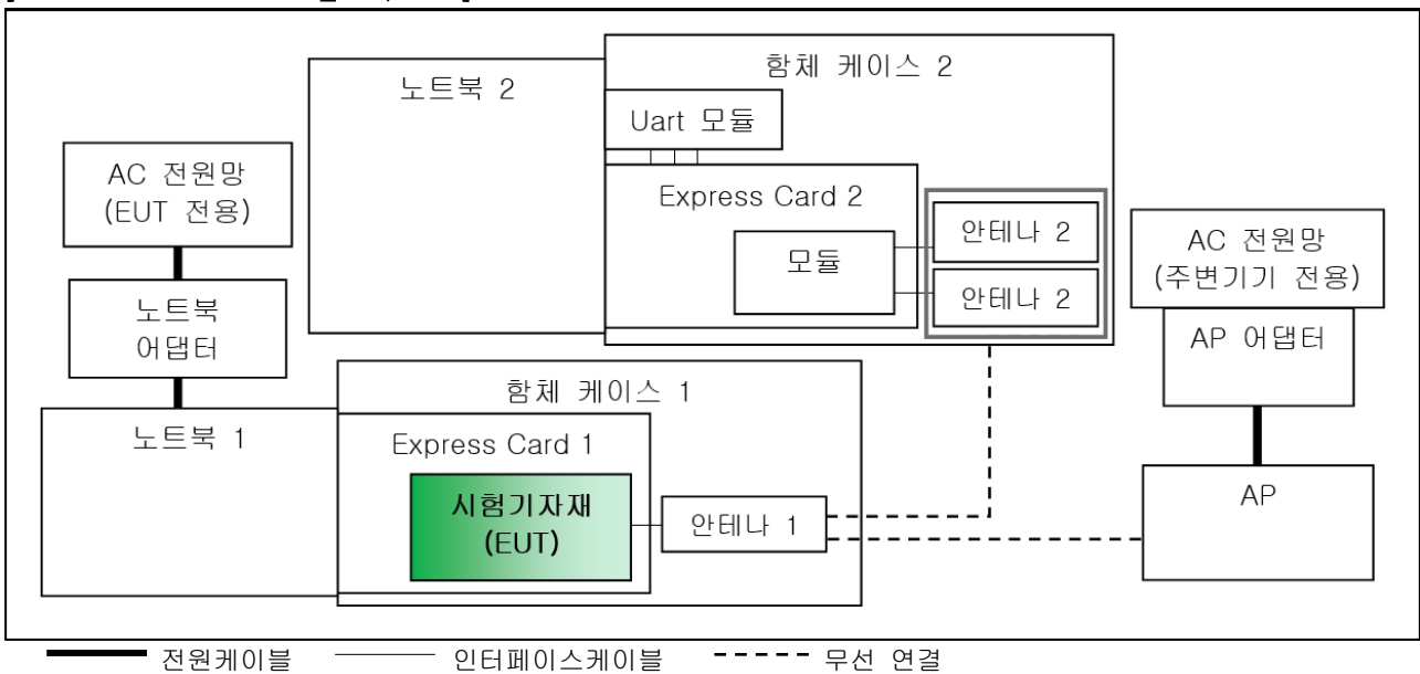
[BT&Wi-Fi 5 GHz 모드_EMI/EMS]
