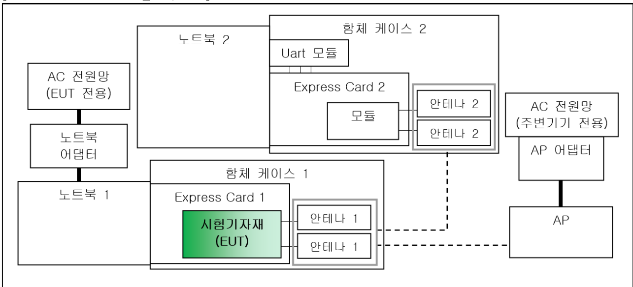
[BT&Wi-Fi 5 GHz 모드_EMI/EMS]
