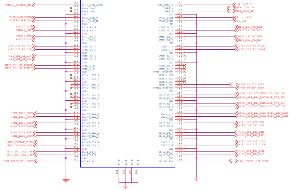
U338 connector_2
